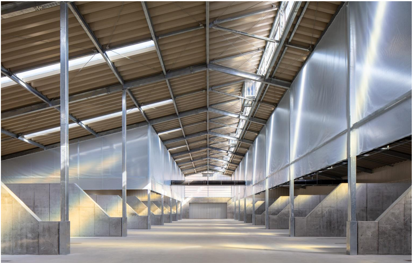
第3期工場 竣工写真(発酵槽)
